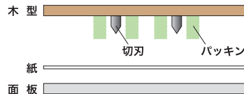
○トムソン木型（打ち抜く版のイメージ）
